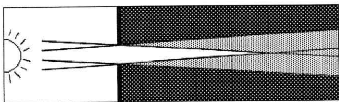
Fig. 4. De grootte van de zonneschijf veroorzaakt een verbreding en vervaging van de lichtstreep die door een smalle verticale spleet valt (bovenaanzicht). De lijnen geven de stralen van de linker en rechter rand van de zon aan (de hoek is overdreven voorgesteld).
